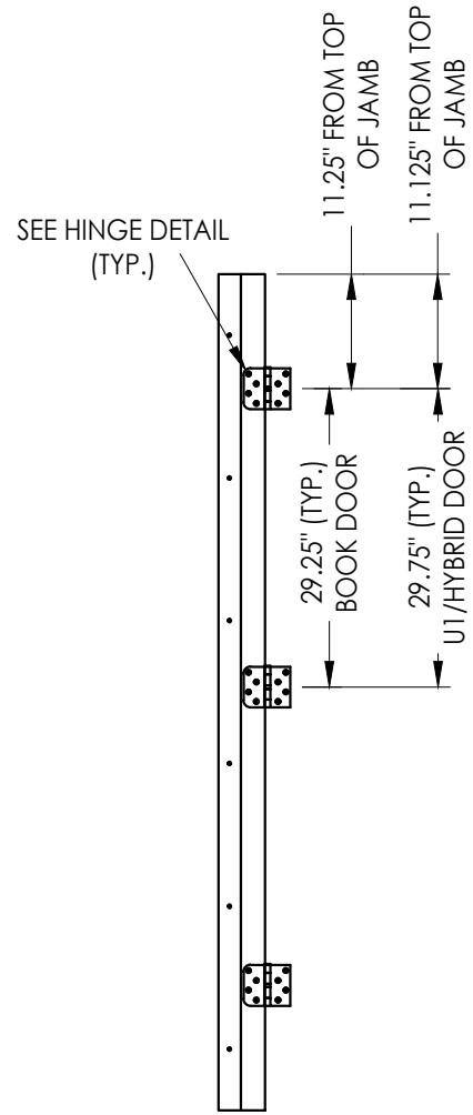
HINGE JAMB
